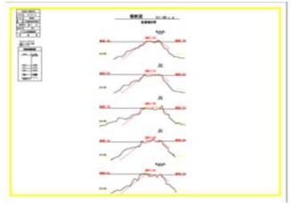
UAV飛行測量による横断面
