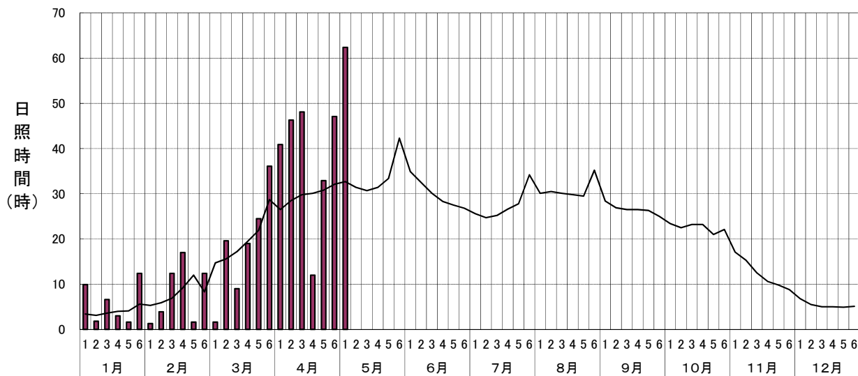
半旬別気象図 日照時間(五所川原:2024年)
