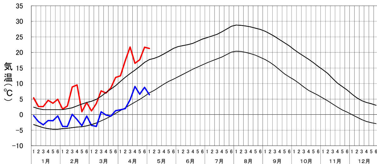
半旬別気象図 最高気温・最低気温(五所川原:2024年)
